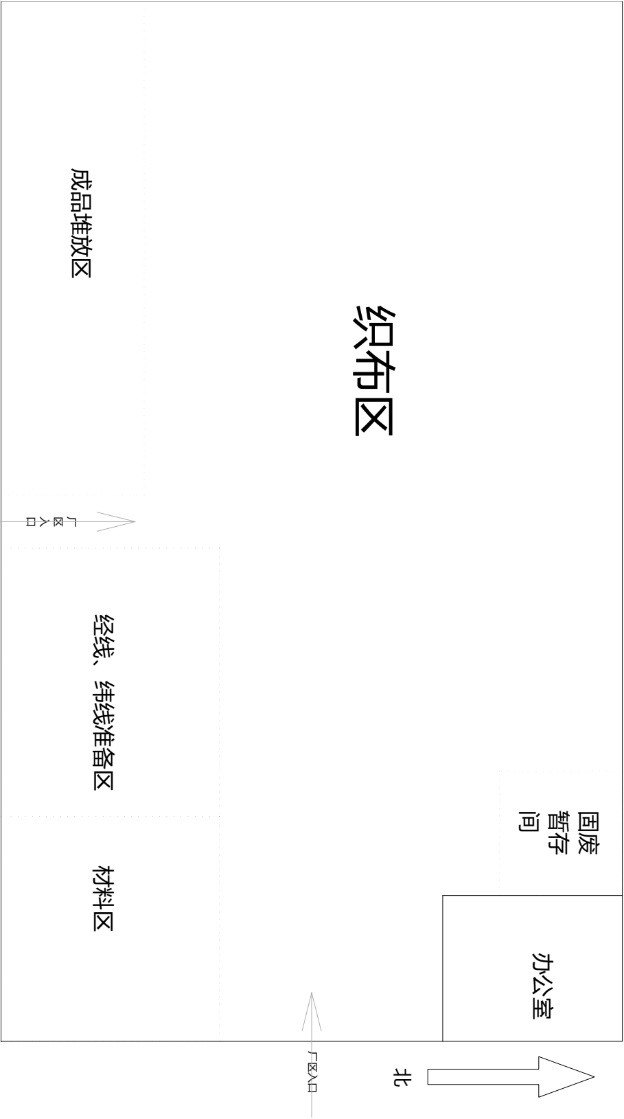
附图4 项目平面布置图
