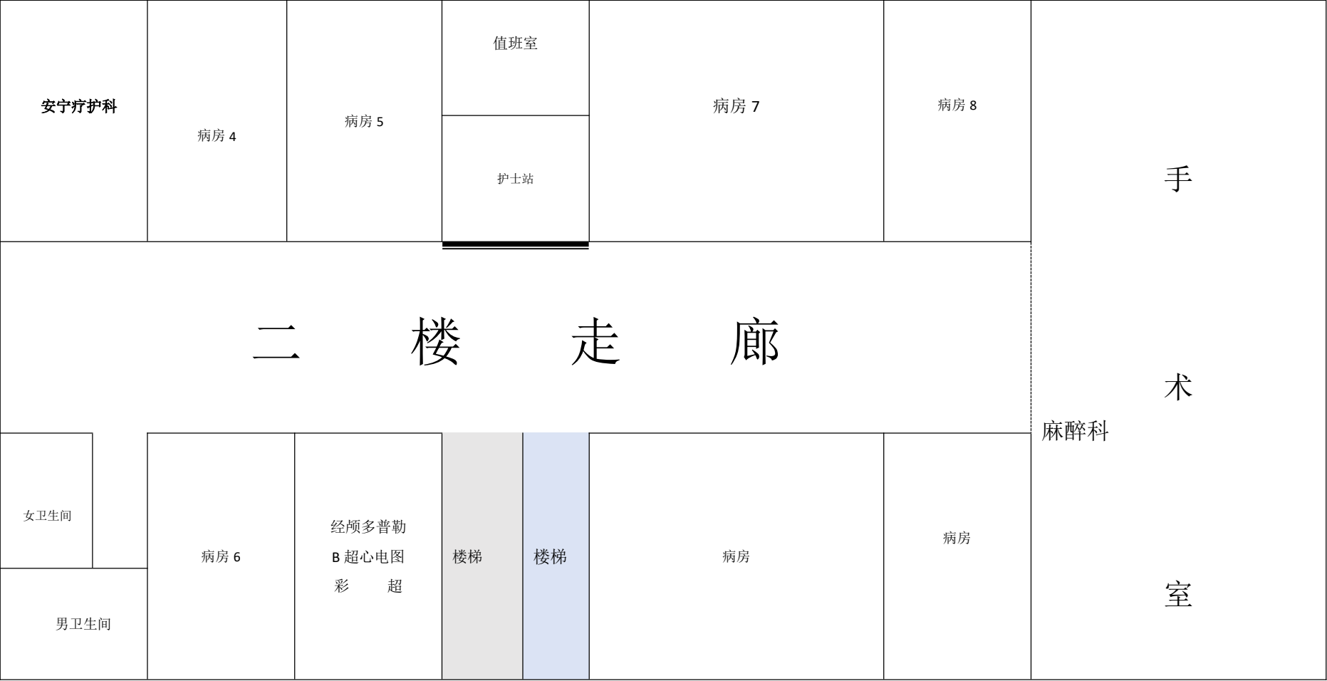
附图 3-2 项目门诊楼二楼平面布置图
