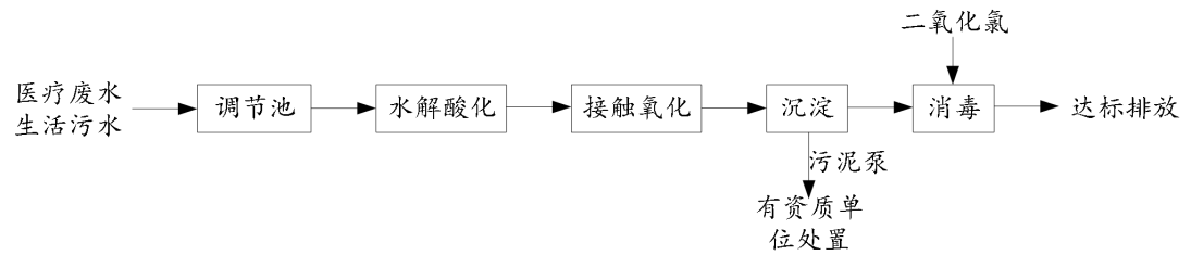
图2 本项目废水处理工艺流程图
