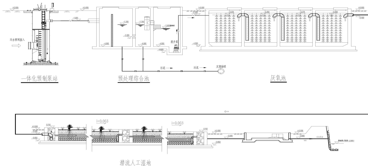
工艺高程流程图
