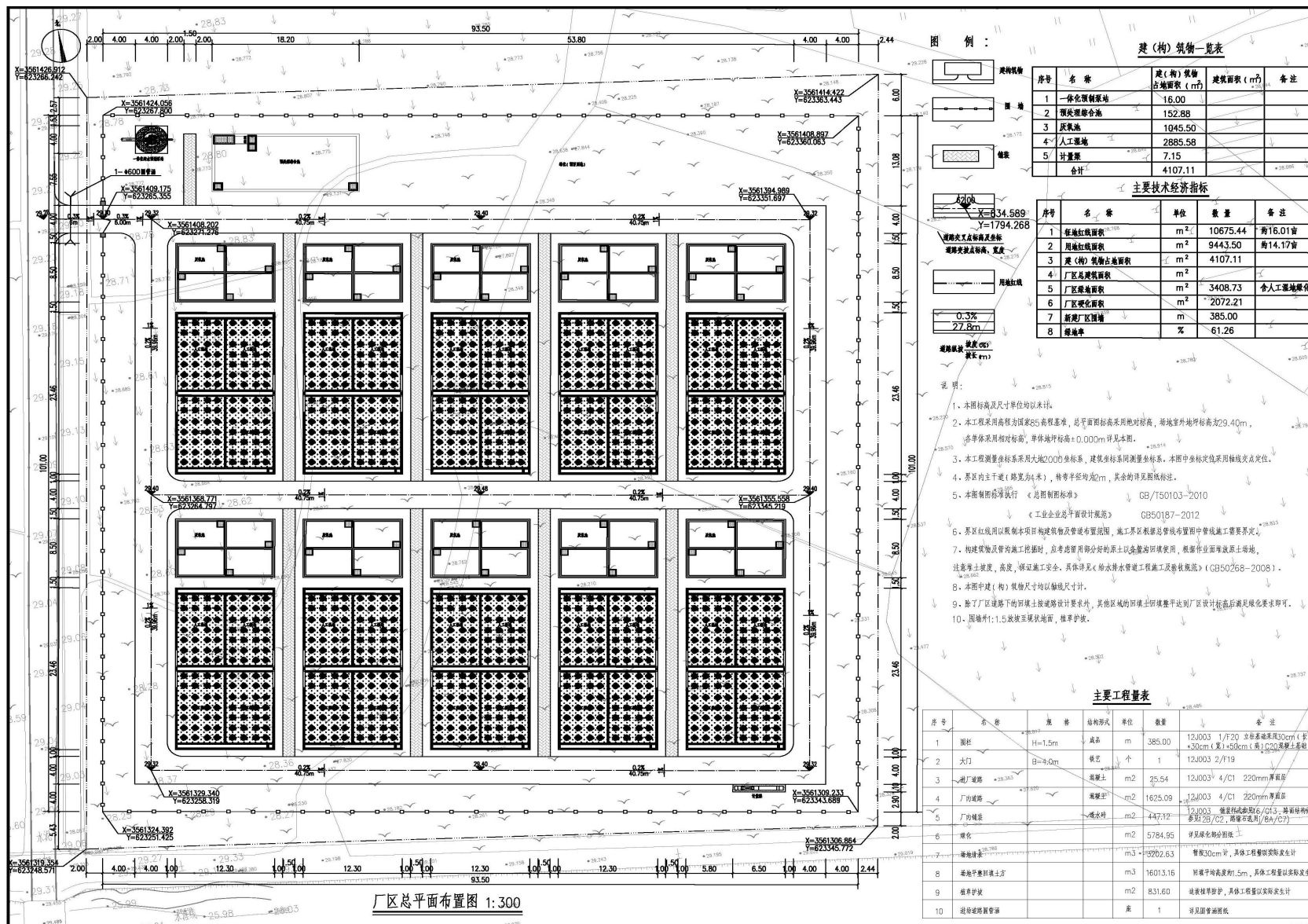
附图 2 污水处理厂总平面布置图
