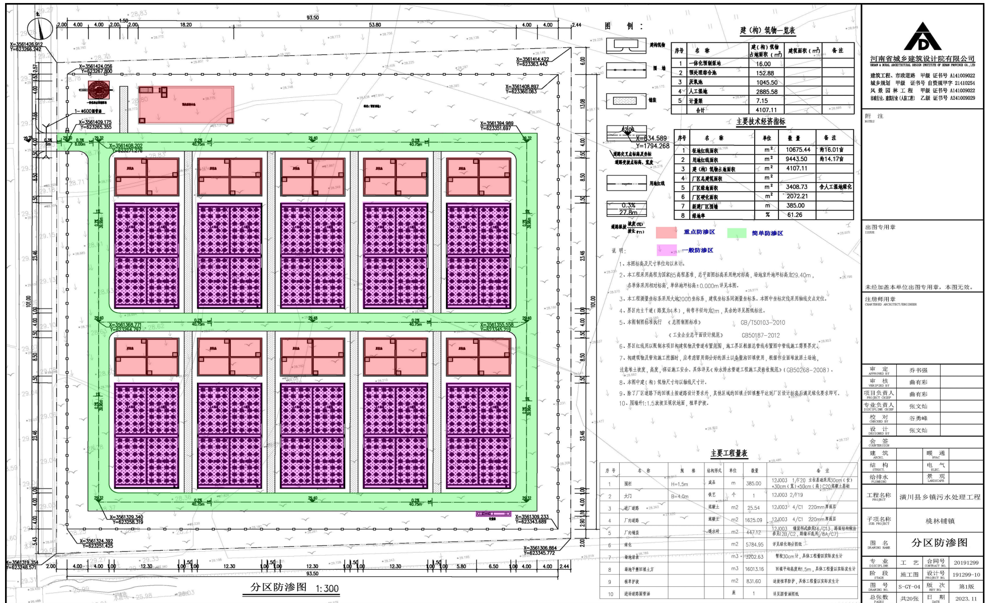
附图 5 分区防渗图
