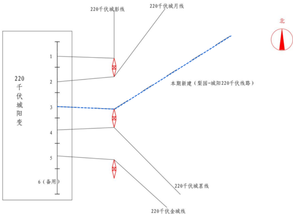
图 3 本期城阳变 220kV 出线间隔示意图
