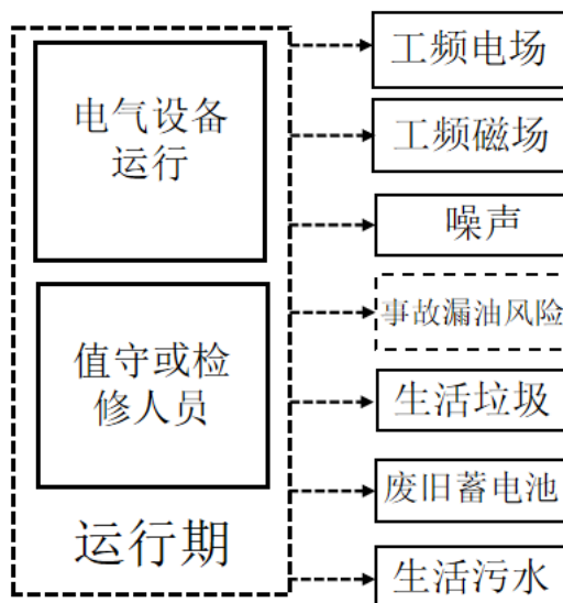
图 9 本工程变电站运行期产污节点图
