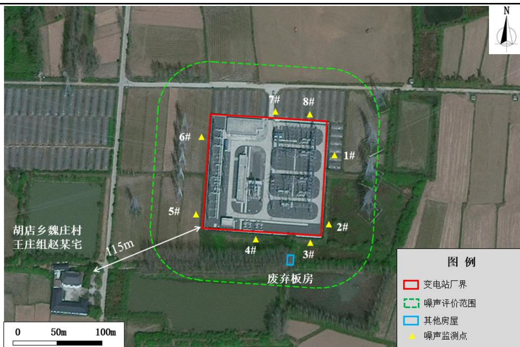
图 7 城阳 220kV 变电站厂界监测布点示意图
