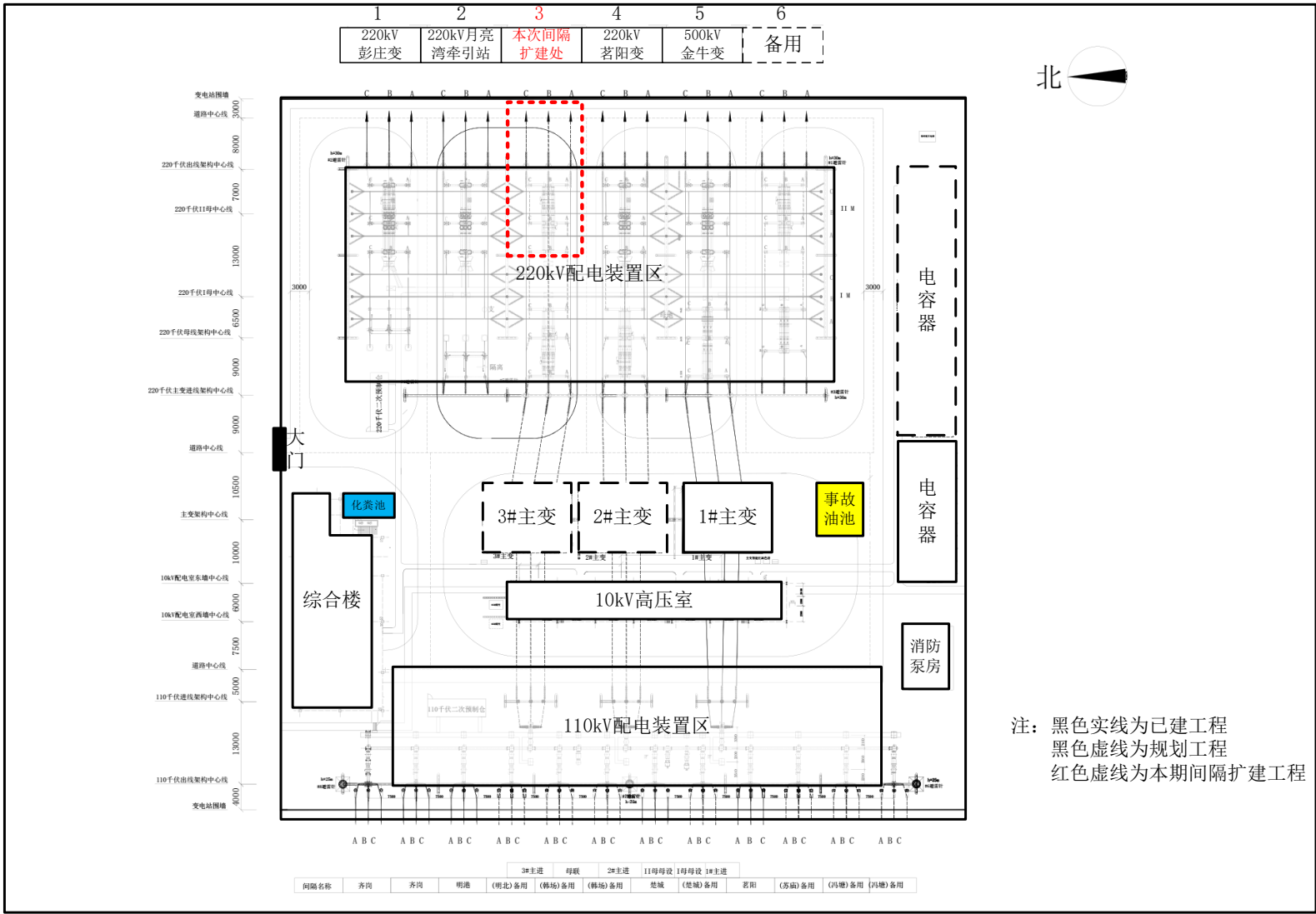
附图 3：城阳 220kV 变电站总平面布置图
