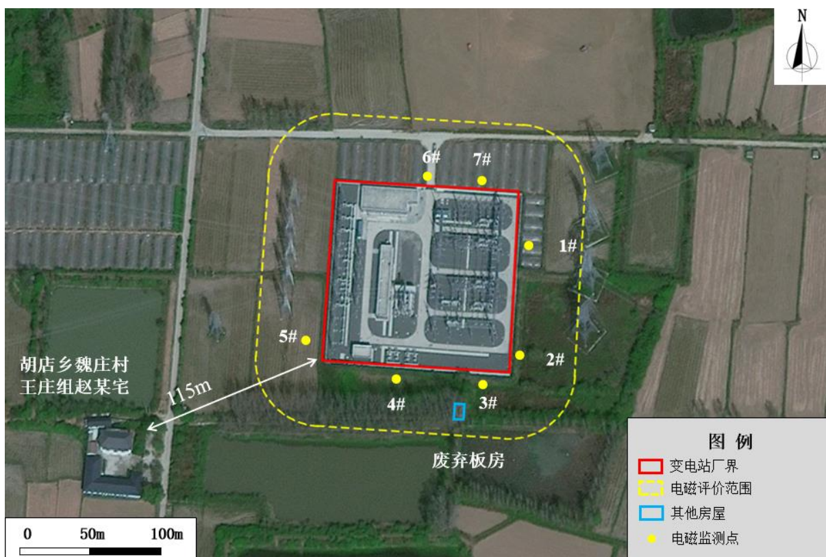
图 10 城阳 220kV 变电站厂界监测布点示意图
