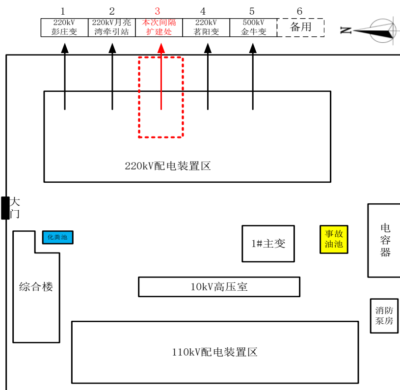
图 4 城阳 220kV 变电站总平面布置示意图
