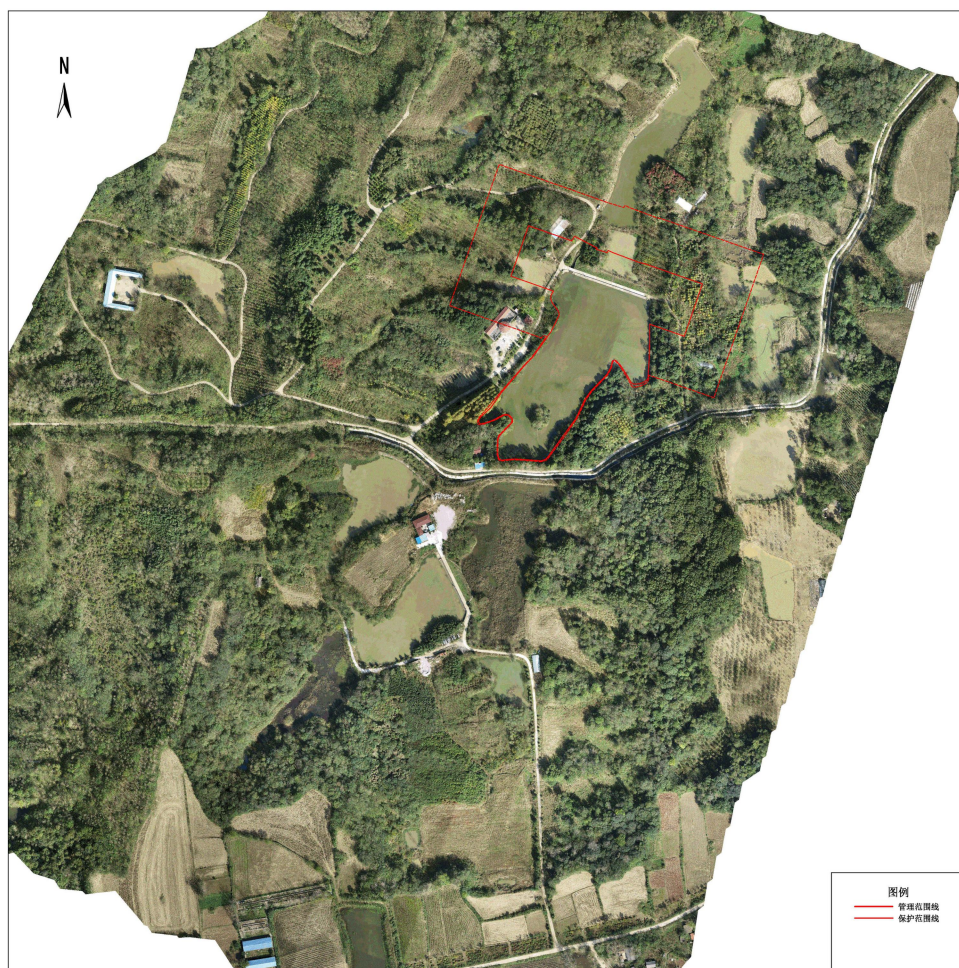
龙井乡连胜水库管理与保护范围公示图
