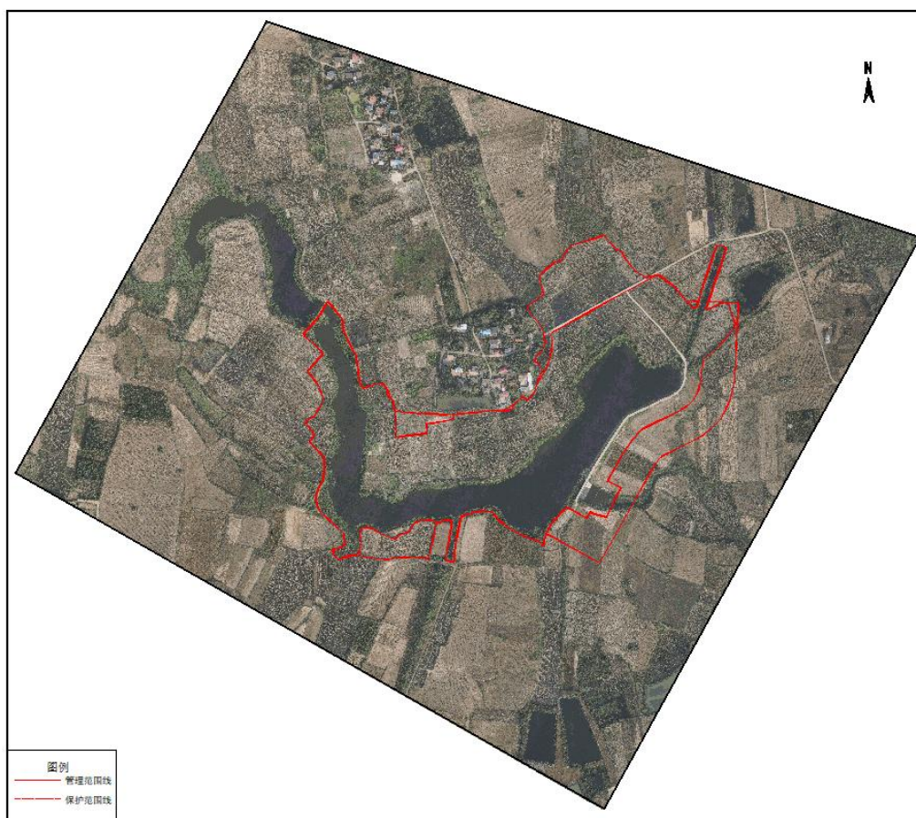
明港镇瓜子桥水库管理与保护范围公示图
