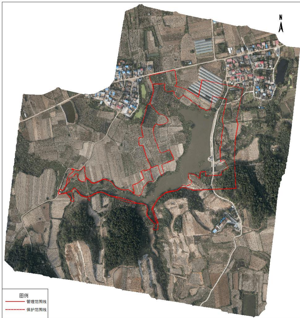
明港镇瓦房庄水库管理与保护范围公示图
