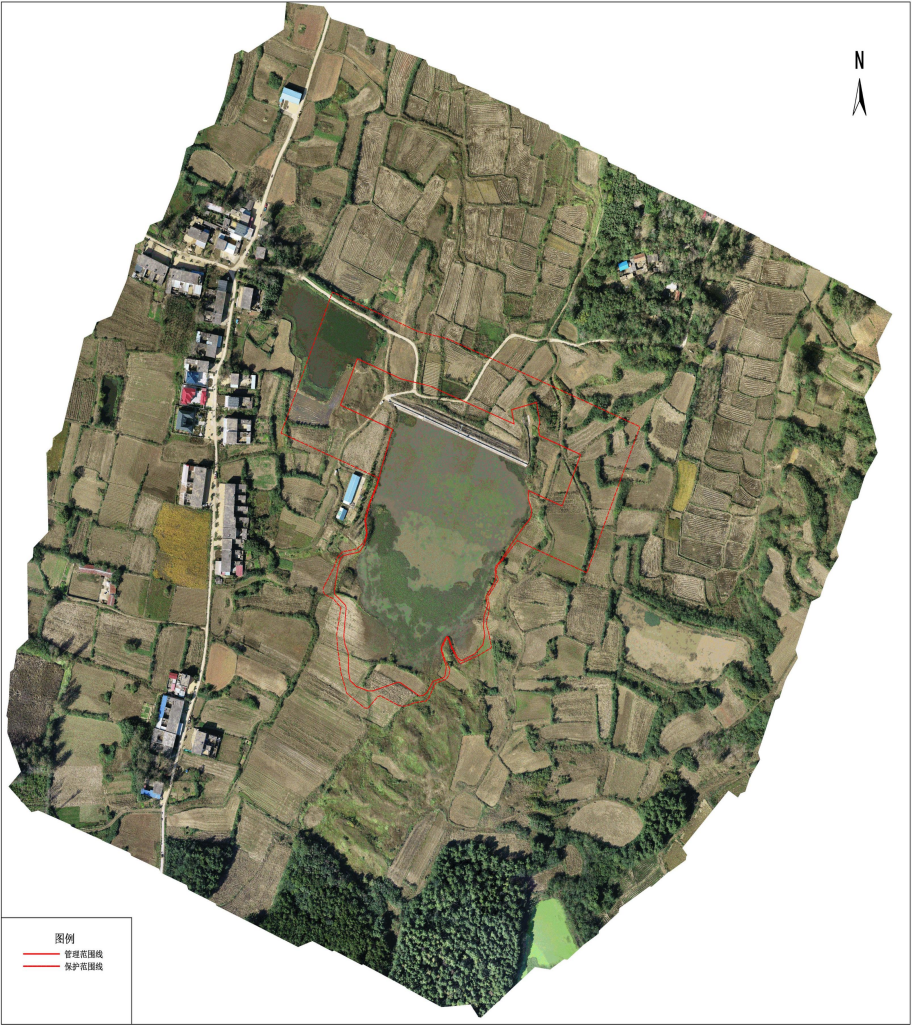
查山乡汤南水库管理与保护范围公示图
