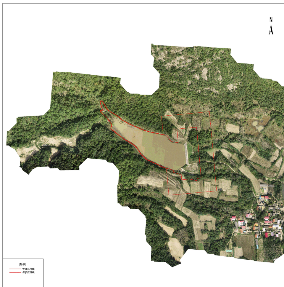
邢集镇上肖楼水库管理与保护范围公示图
