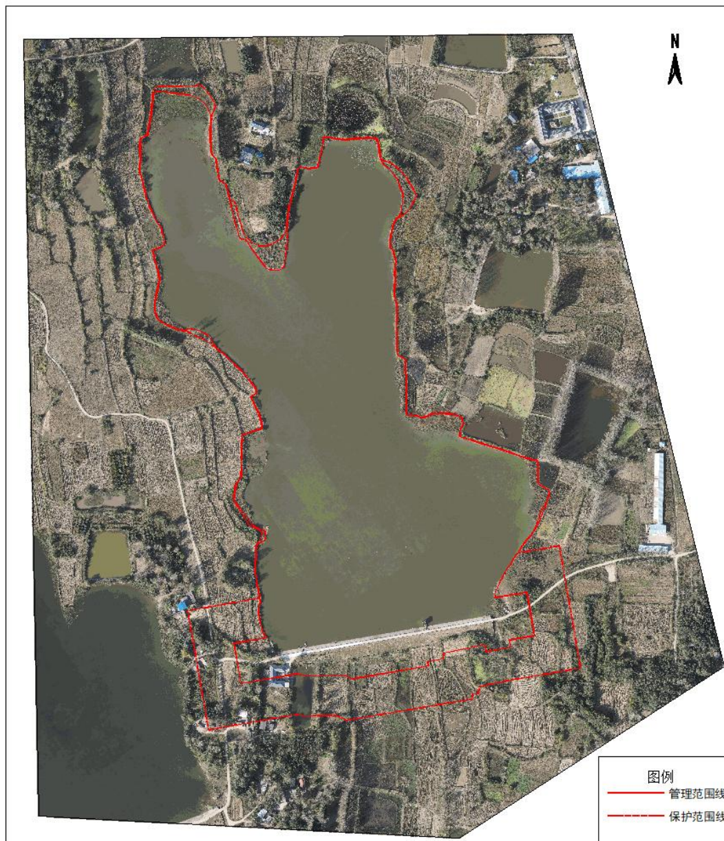
洋河镇姚冲水库管理与保护范围公示图
