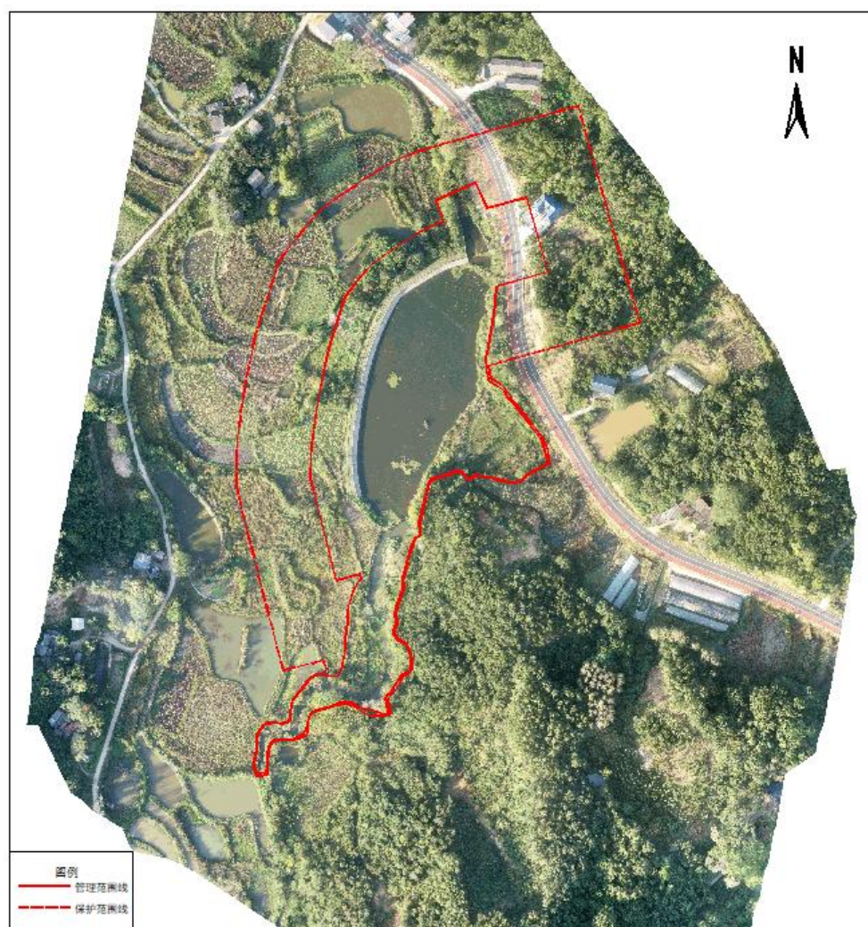
五里店街道办事处红庙水库管理与保护范围公示图
