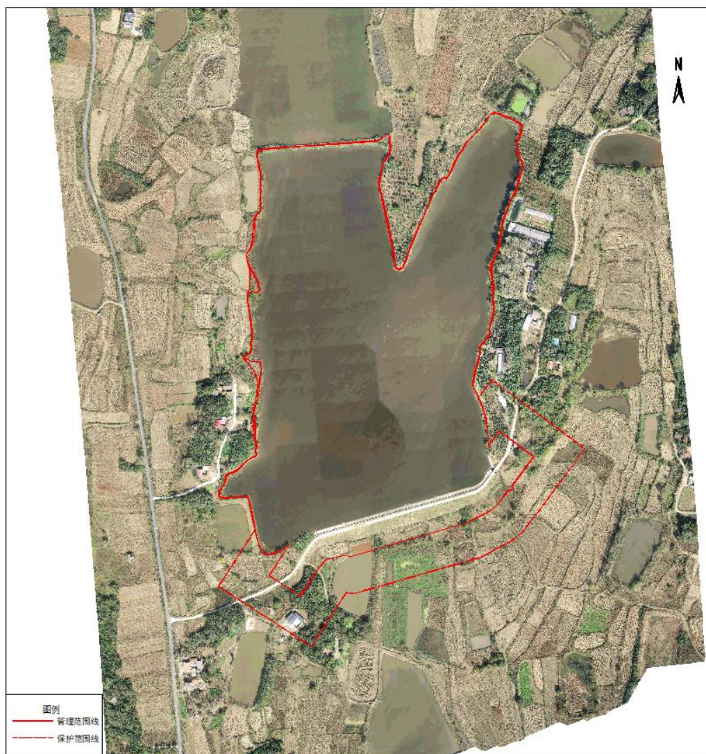
洋河镇董冲水库管理与保护范围公示图
