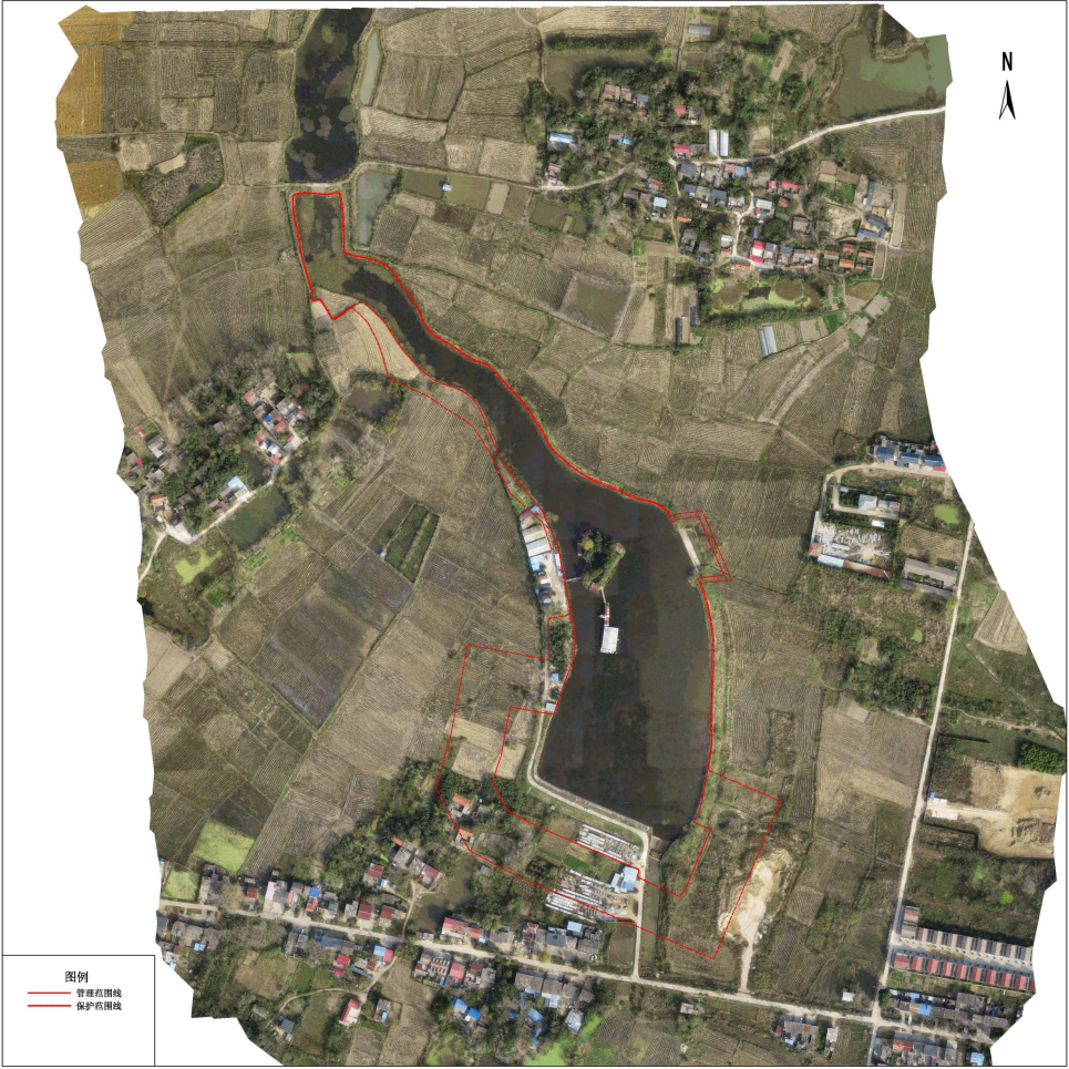
甘岸办事处冯堰水库管理与保护范围线公示图
