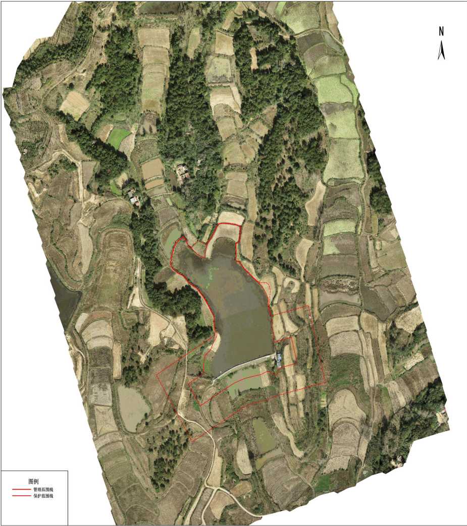
高粱店乡王家大堰水库管理与保护范围公示图
