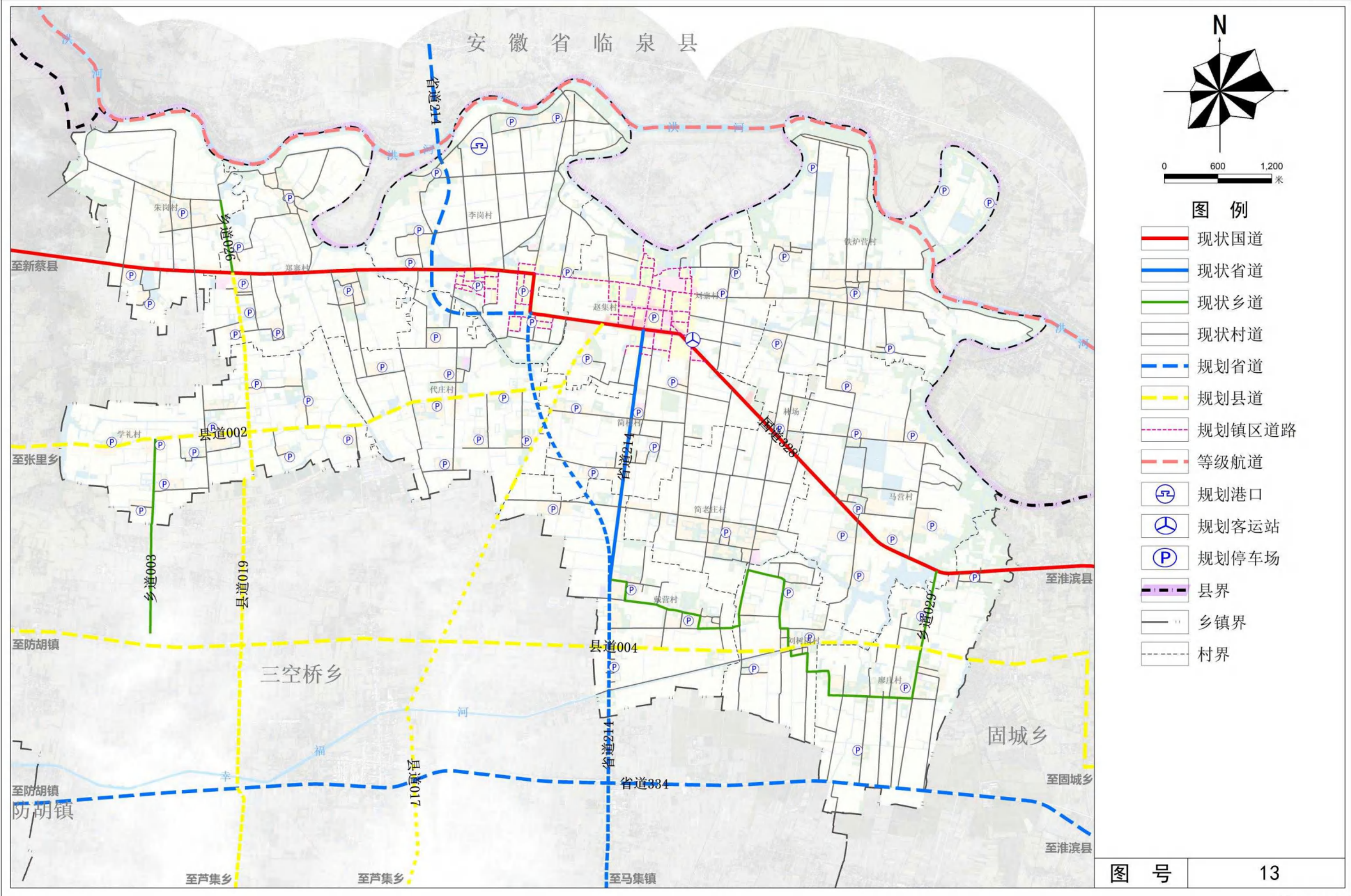
镇域综合交通规划图
