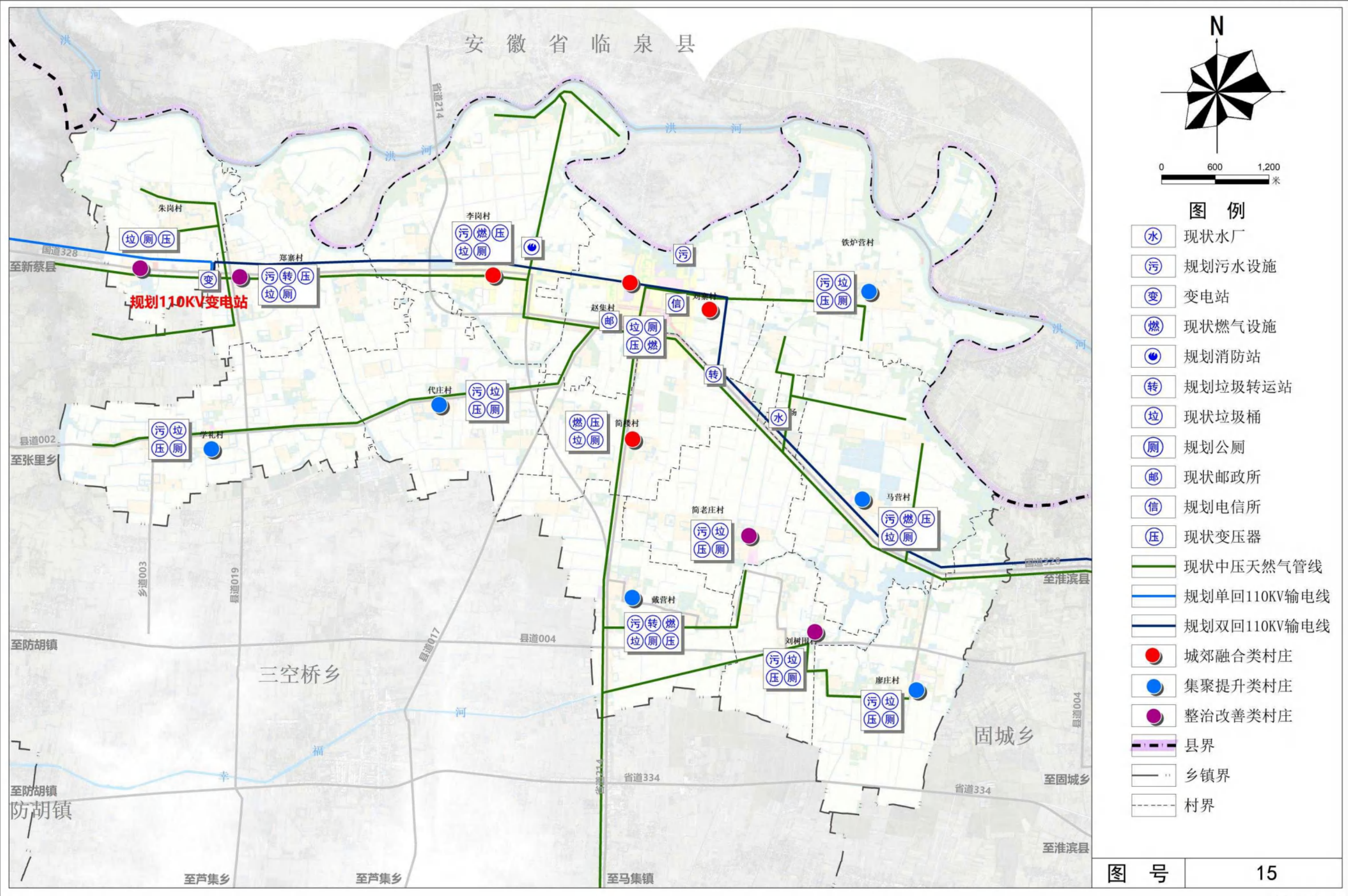
镇域基础设施规划图
