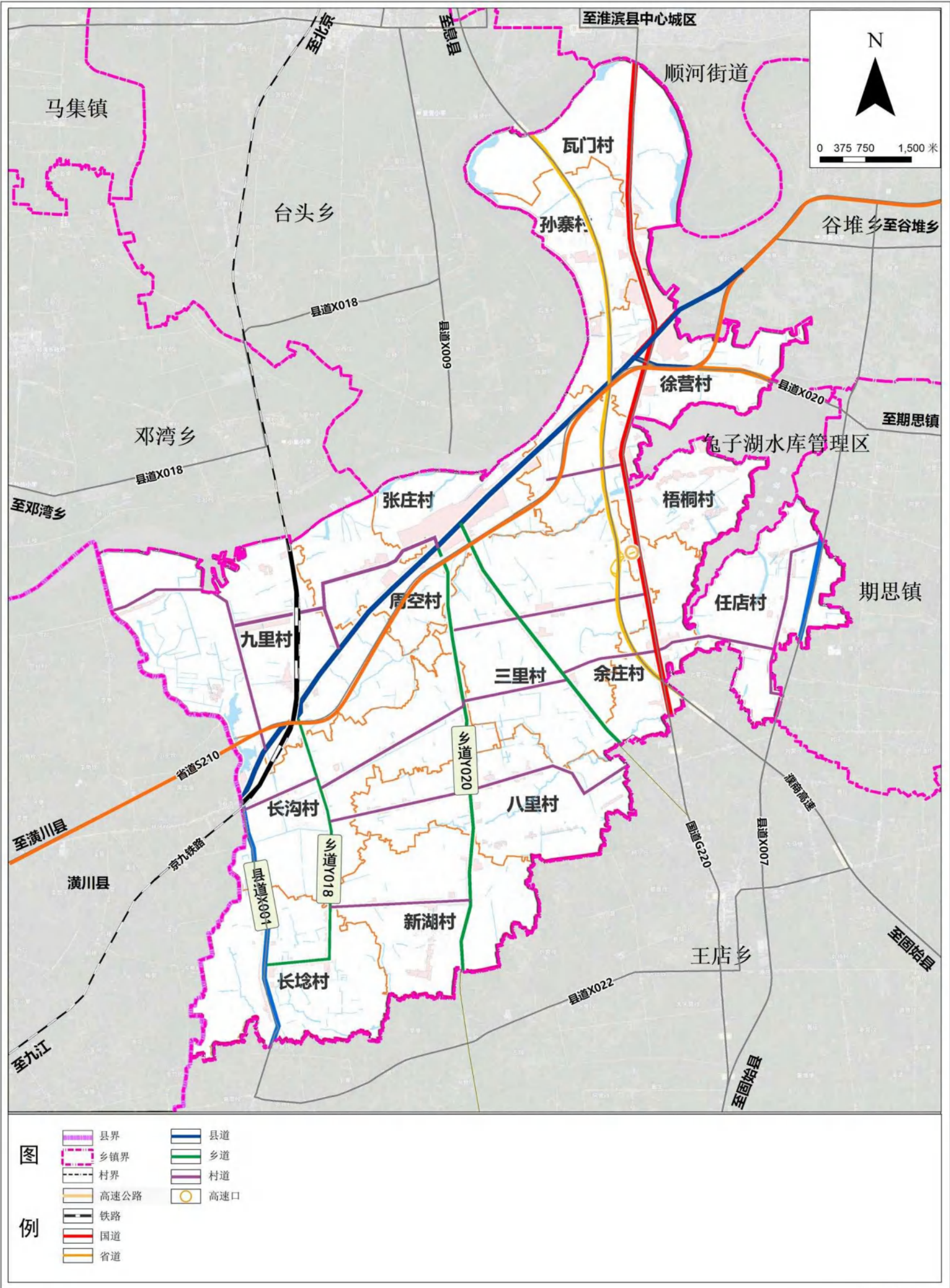
乡域综合交通规划图
