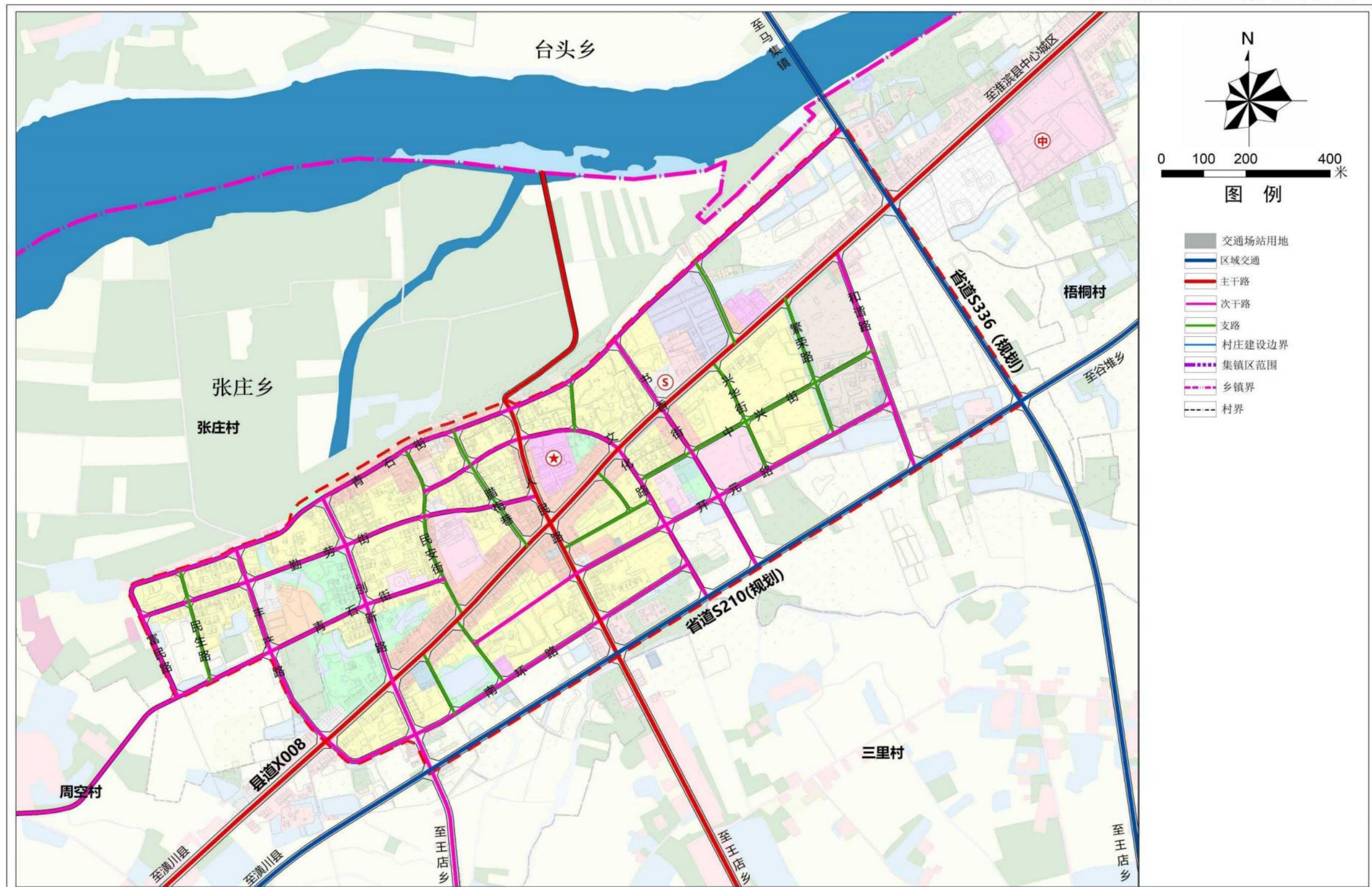
乡政府驻地道路交通规划图
