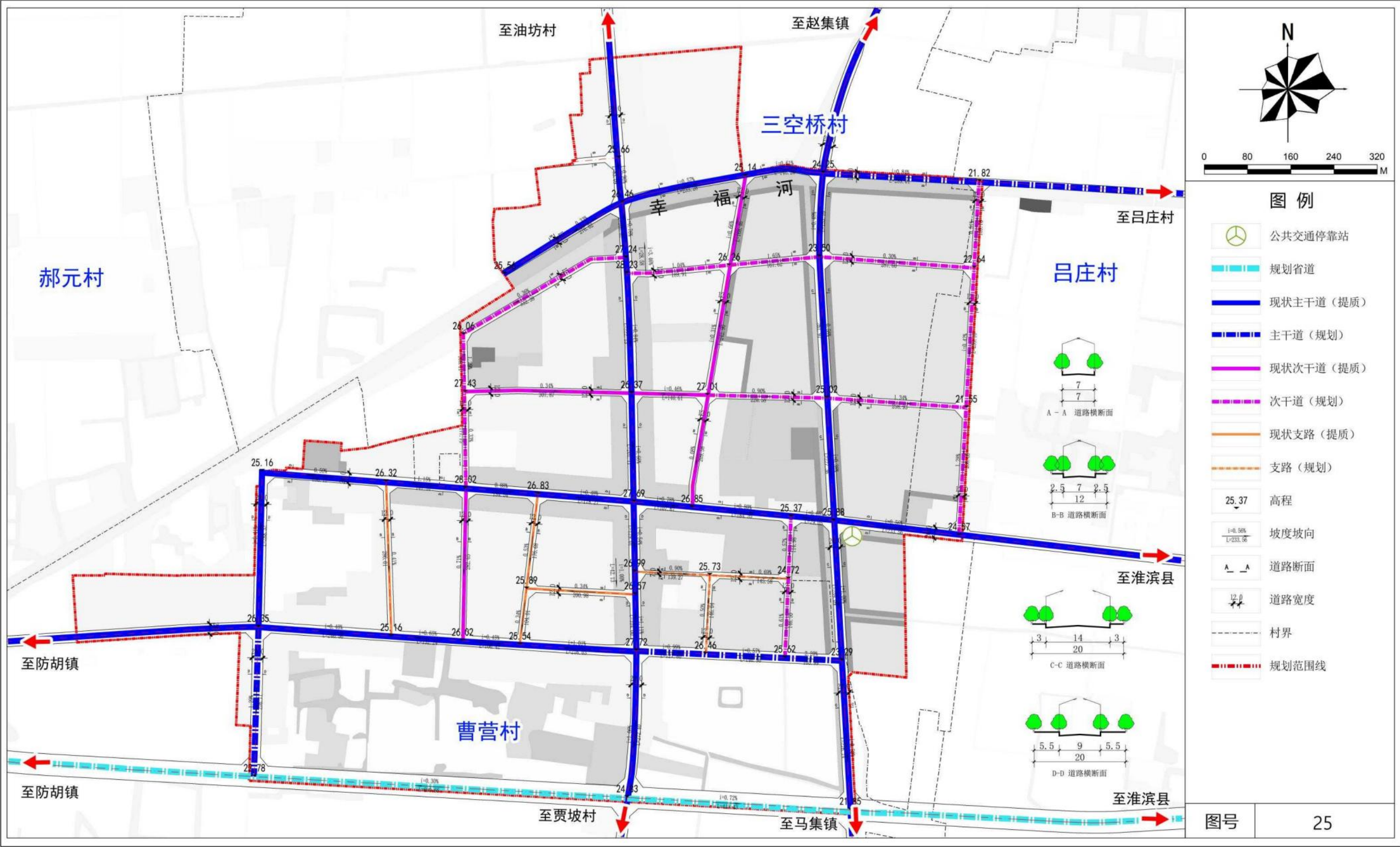
乡政府驻地道路交通规划图
