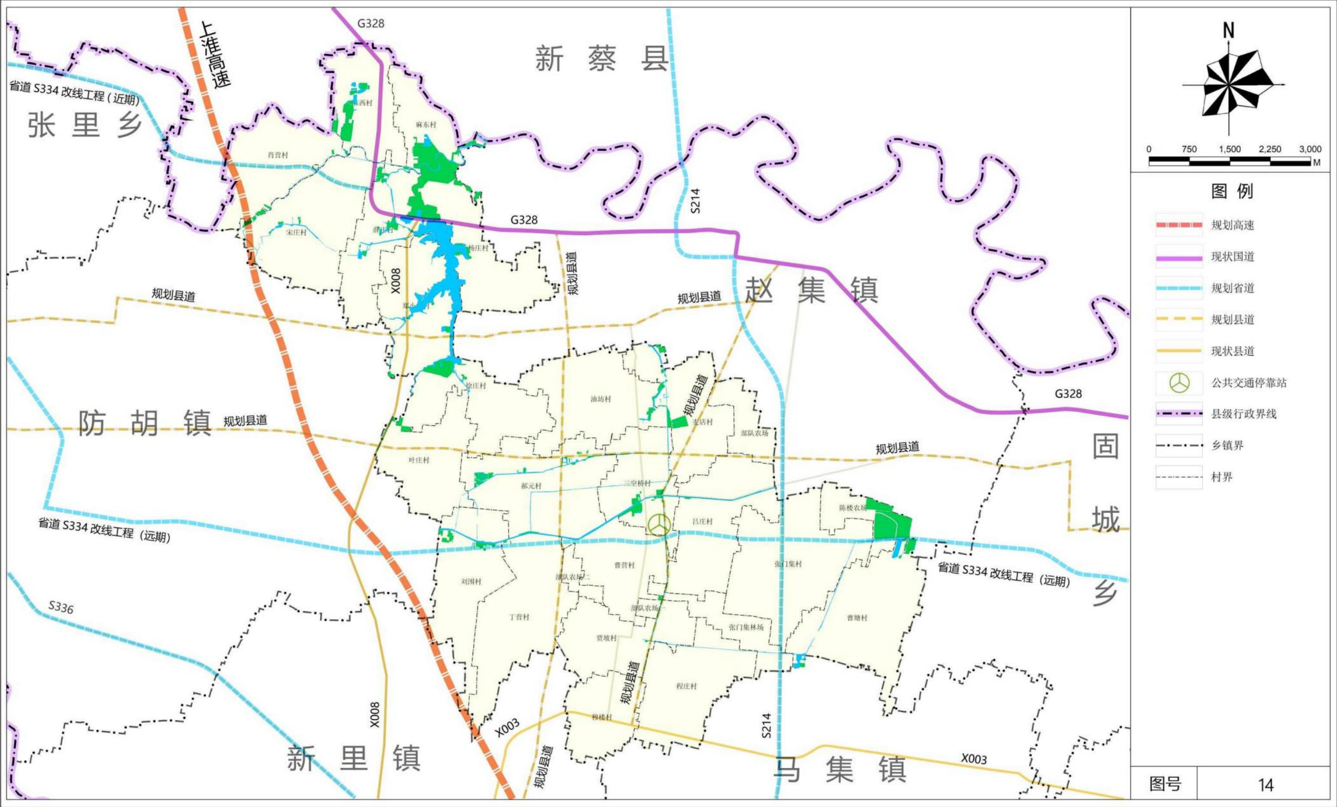
乡域综合交通规划图
