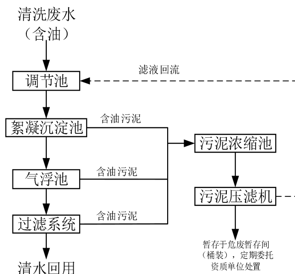
图3 厂区污水处理站工艺流程图
